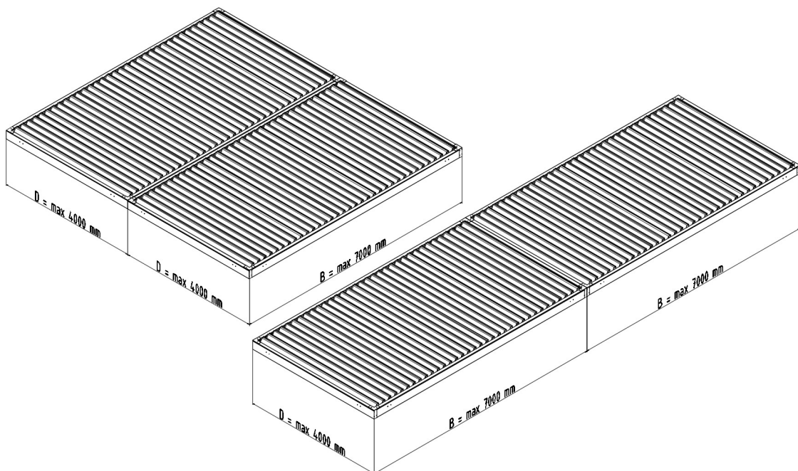
Zeichn. 2. Pergola SB 400 PRO R Längs- oder Querverbindung – durch die Quer- oder Seitenstreben
