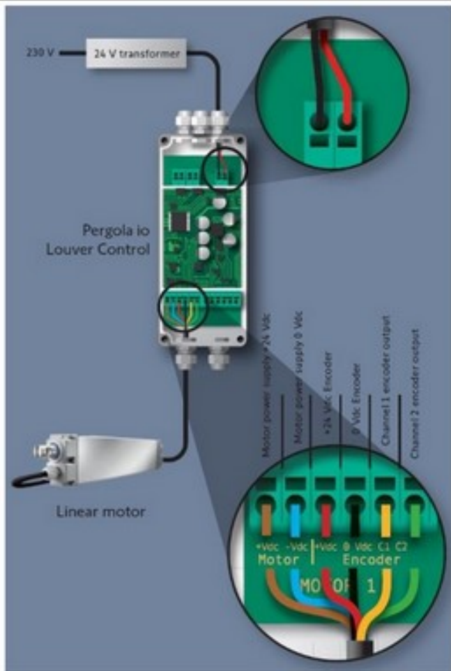
Zeichn. 35 Anschlussdiagramm im Funkempfänger Pergola io Louver
