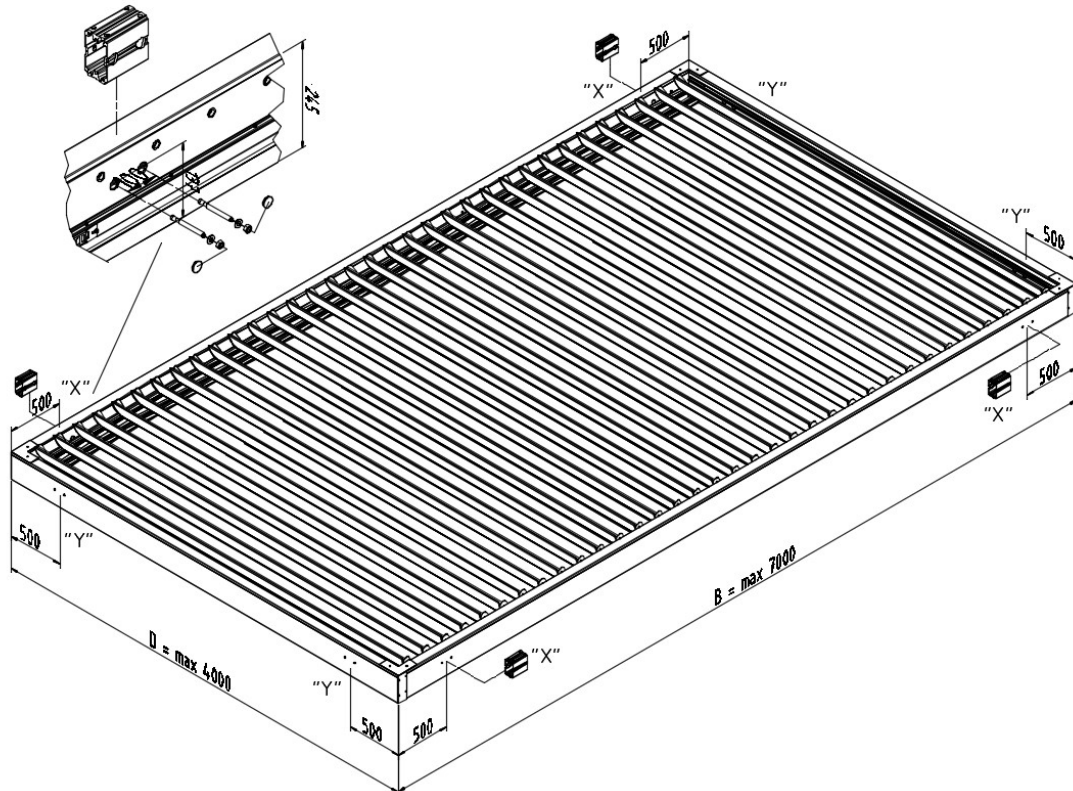
Zeichn. 4. Empfohlene Verankerungspunkte („X“ -an den Seitenstreben - alternativ „Y“ an den Querstreben)
