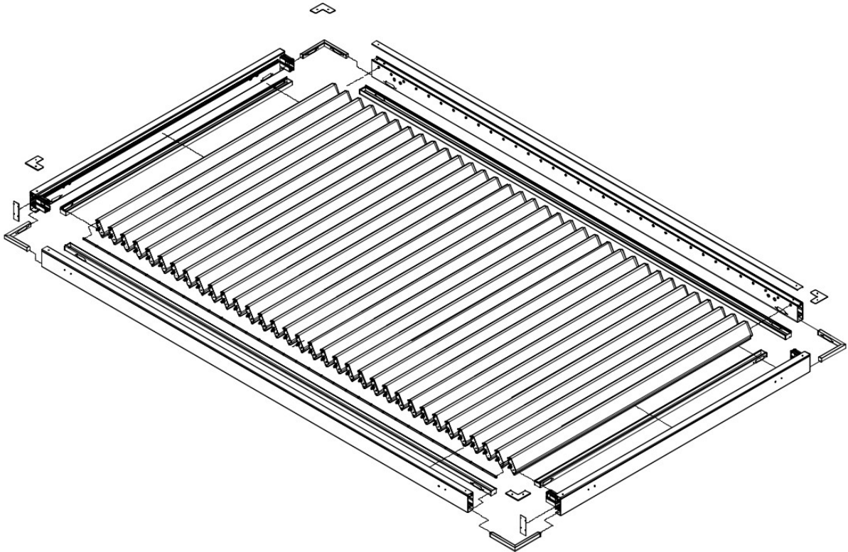
Zeichn. 7. Montageansicht der Pergola SB 400 PRO R- mit 4 Regenrinnen
