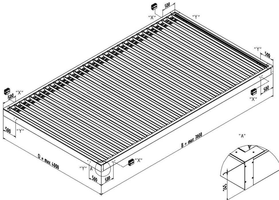
Zeichn. 1. Pergola SB 400 PRO R - Abmessungen: B max – max. Ausladung, D max – max. Breite, H – Höhe (245 mm + 3mm Eckabdeckkappe), Verankerungspunkte durch die Streben - X=Seitenstreben, Y=Querstreben
