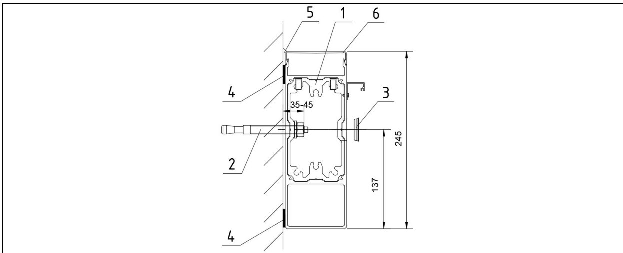
Zeichn. 5 – Verankerung (1- Verstärkung in der Strebe am Verankerungspunkt, 2- Anker M12 (nicht im Lieferumfang enthalten), 3-beschichtete Abdeckkappe, 4-EPDM-Streifen, 5-mit Dichtmittel abdichten, 6- Strebenrevision).
