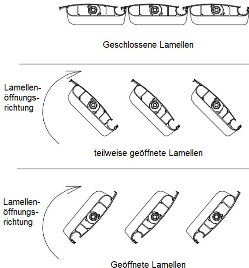
Zeichn. 3. Standardöffnungsrichtung der Lamellen der Pergola SB 400 PRO R.
