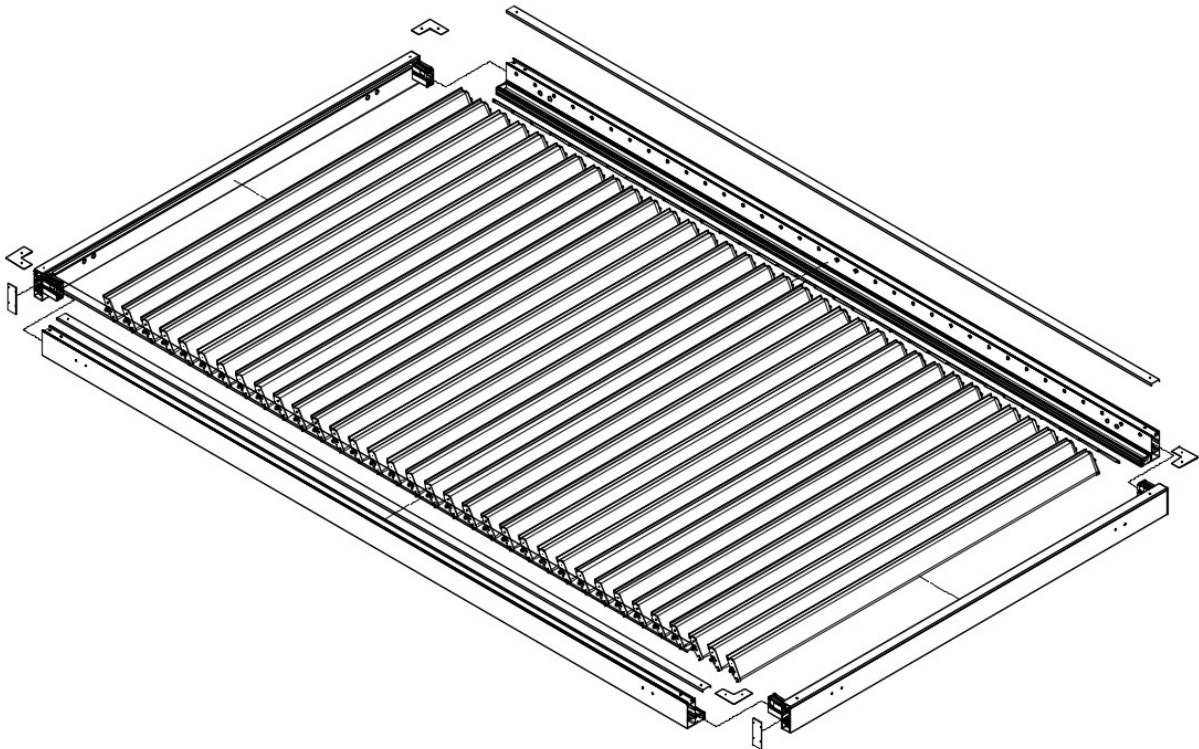
Zeichn. 6. Montageansicht der Pergola SB 400 PRO R- mit 2 Regenrinnen
